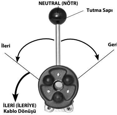
Şekil 14 – AUTOFEED Kablo Besleme Yönleri (Makinenin Önünden Görüntülenen)
