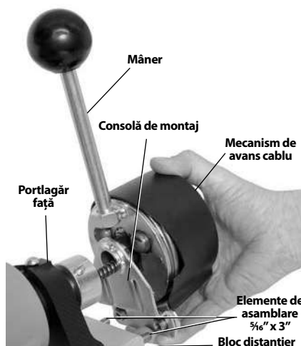
Figura 5 – Montarea mecanismului de avans cablu pe cadru
