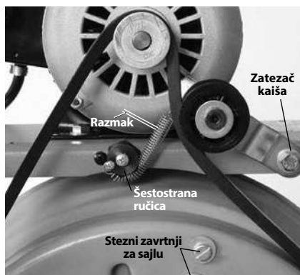
Slika 17 – Graničnik podešavanja obrtnog momenta. (Prikazano sa skinutim zaštitnim kaišem)
