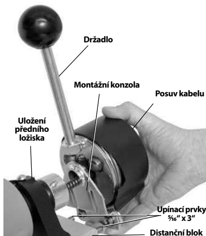
Obrázek 5 – Montáž posuvu kabelu na rám
