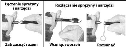
Rys. 12 – Podłączanie/odłączanie narzędzi
