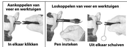
Figuur 12 – Werktuigen bevestigen/loskoppelen
