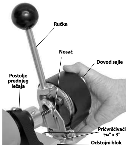
Slika 5 – Montaža dovoda sajle na ram
