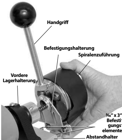
Abbildung 5 – Anbringen der Spiralenzuführung am Rahmen
