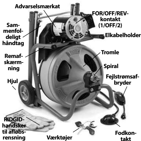
Figur 1 – K-400-tromlemaskine
