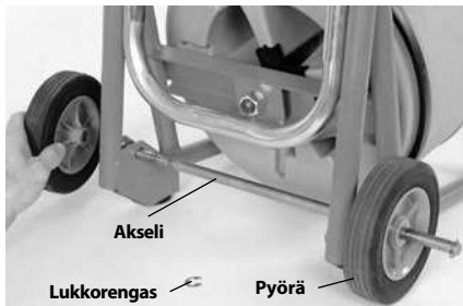
Kuva 4 – Pyörän asentaminen
