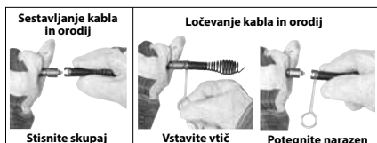
Slika 12 – Povezovanje/odklapljanje orodij
