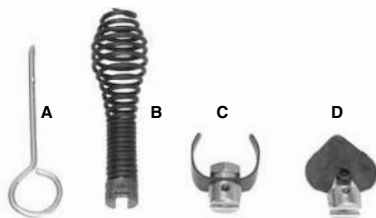
Figure 11 – Outils de curage fournis avec le K-400
