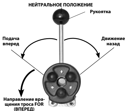
Рис. 14 – Направления подачи троса с помощью механизма AUTOFEED (если смотреть с передней стороны машины)
