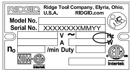
2-сурет – Құрылғының сериялық нөмірі
