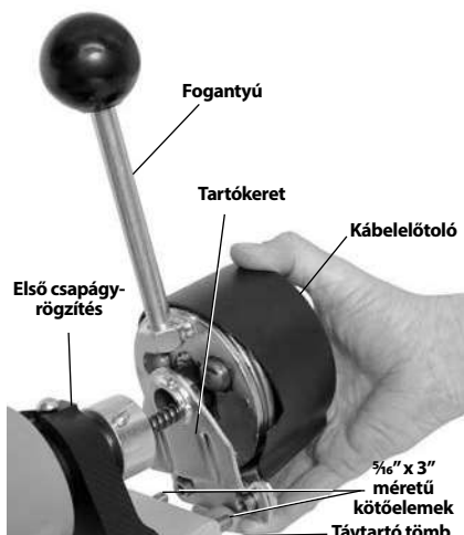
5. Ábra – A kábelelőtőlő felszerelése a vázra
