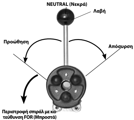
Εικόνα 14 – Κατεύθυνσεις συστήματος τροφοδότησης σπιράλ AUTOFEED (κοιτώντας από το μπροστινό τμήμα του μηχανήματος)
