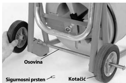
Slika 4 – Sastavljanje kotača
