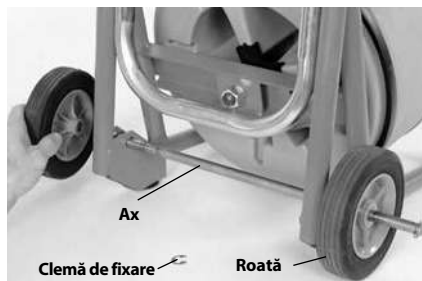
Figura 4 – Asamblare roată
