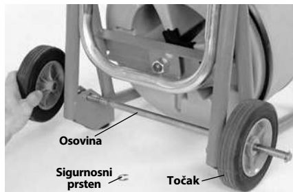
Slika 4 – sastavljanje točka
