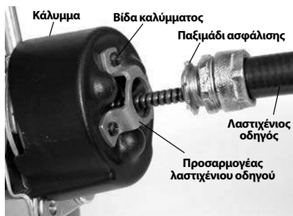
Εικόνα 6 – Τοποθέτηση λαστιχένιου οδηγού στο σύστημα τροφοδότησης σπιδράλ
